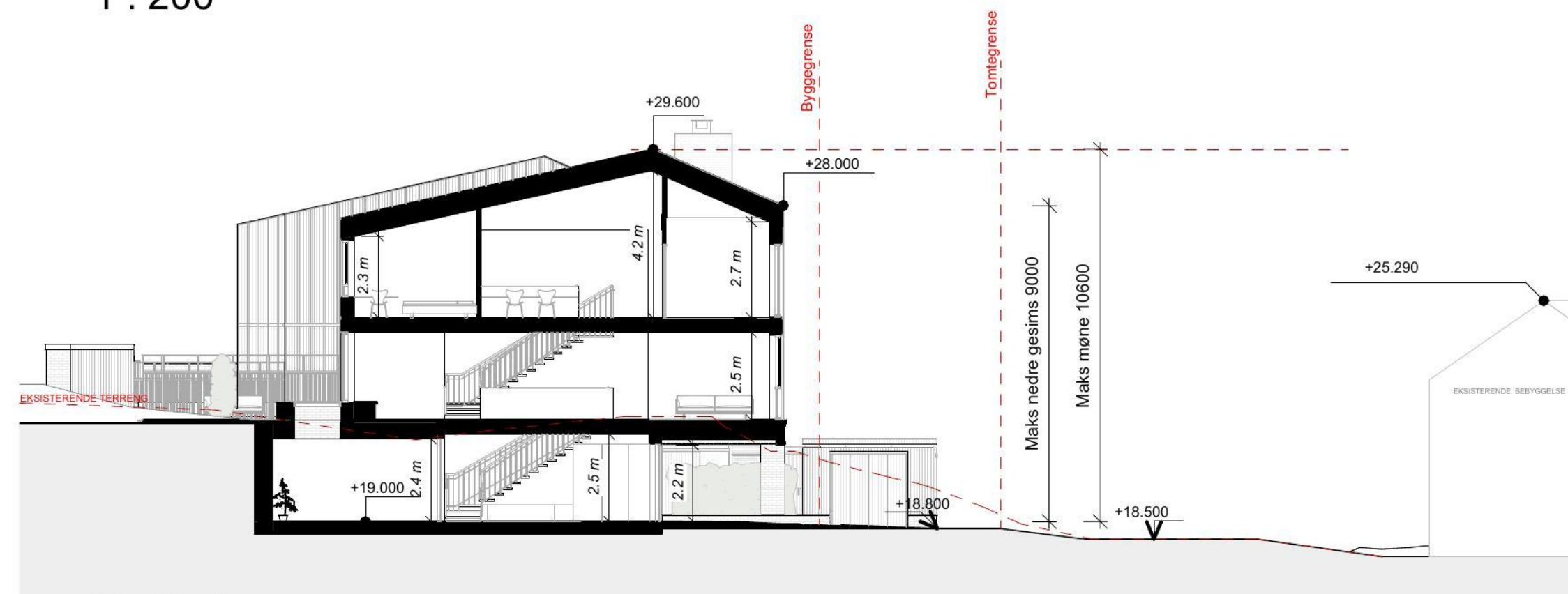
Snitt 1 1 : 200
