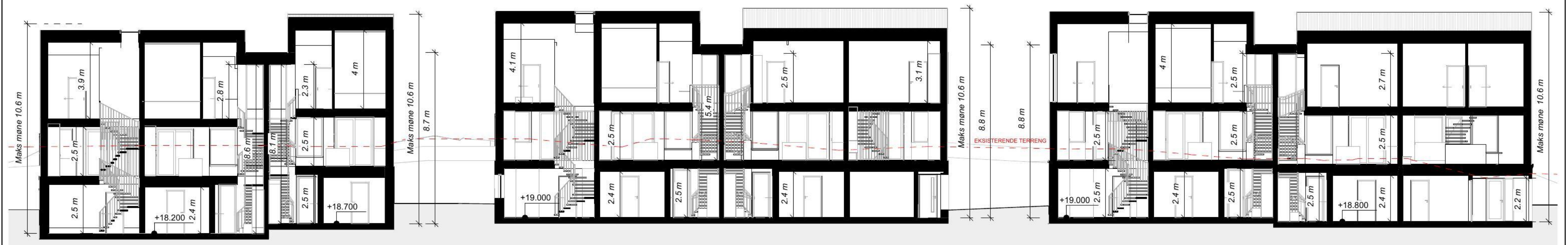
Snitt 2 1 : 200
